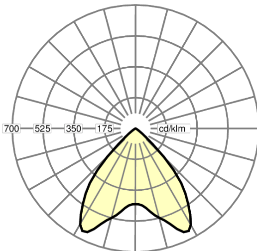
Leveä valonjako (HEIP HRLB)
