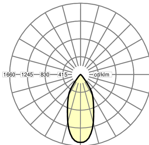
Kapea valonjako (HEIP HRLTB)
